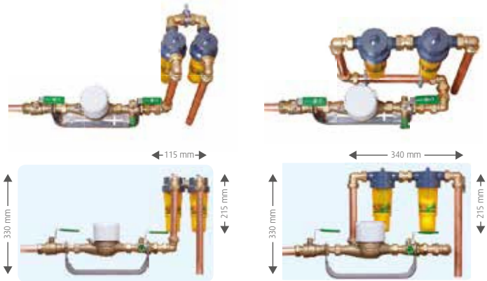
NoCalc PrefilterPLUS
